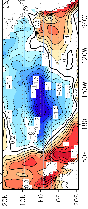
(a) SSTA MAM 2009
